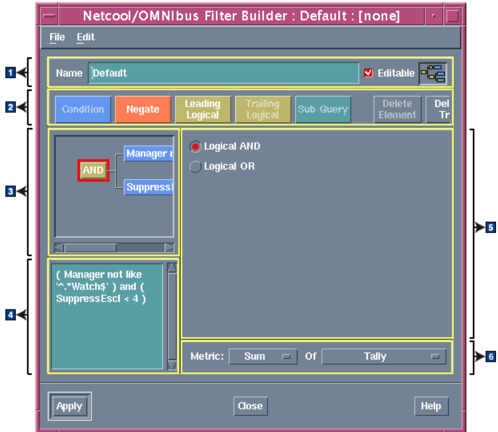
Figure 9. Générateur de filtres sous UNIX
